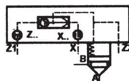
Válvula alternativa
