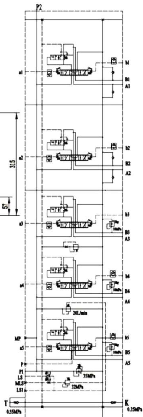
Esquema Hidráulico
