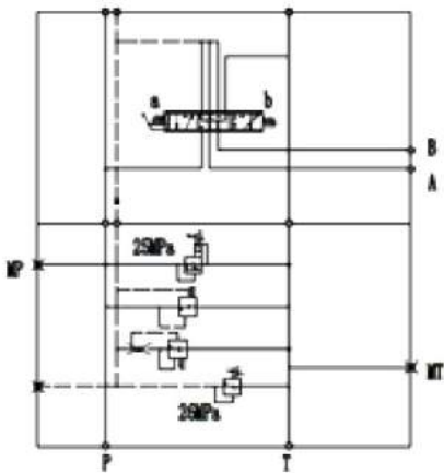
Esquema Hidráulico
