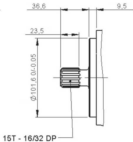
Eje estriado Z15 16/32 DP
