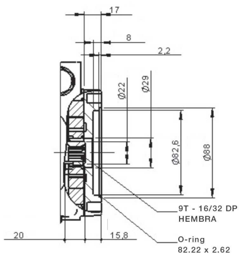
Brida de fijación SAE A
