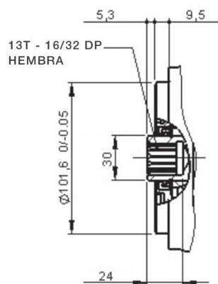
Brida de fijación para bomba TANDEM
