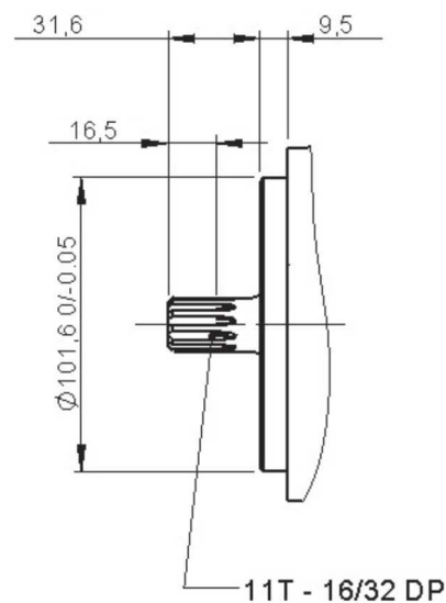
Eje estriado Z11 16/32 DP
