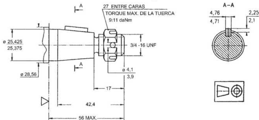
T \varnothing 25,4; SAE J501 cónico con chaveta 3/16" x 3/16" x 3/4" torque máximo 44 daNm
