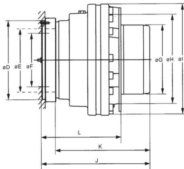
Motor con freno multiplacas
