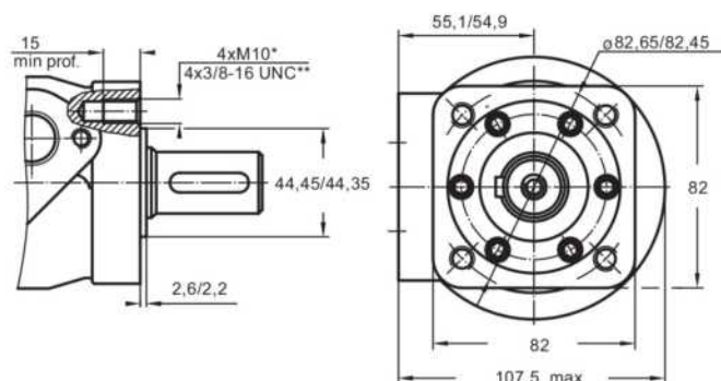
M y Q Brida Cuadrada
