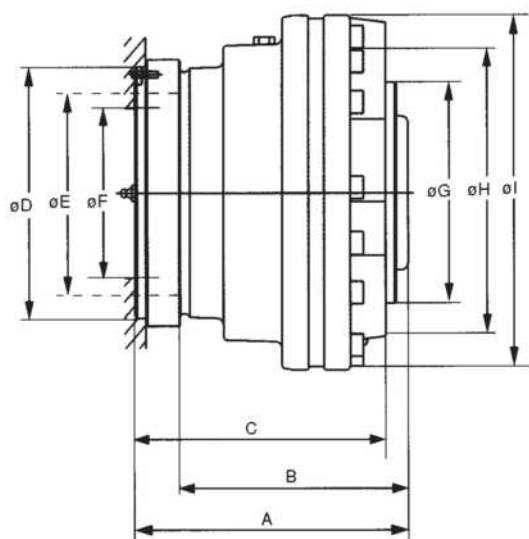
Motor sin freno
