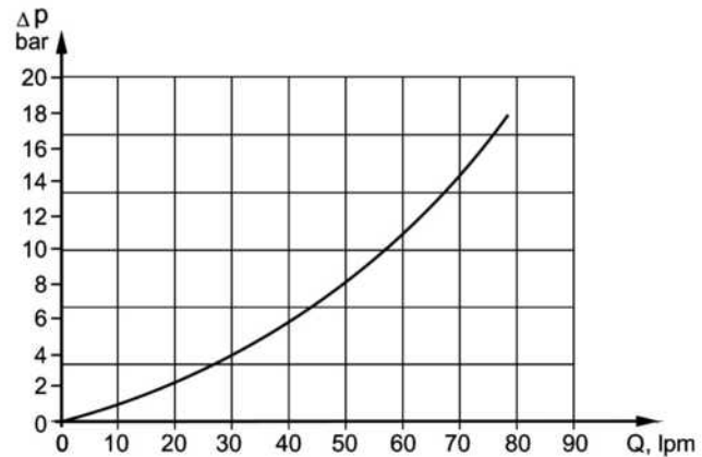
Pérdidas de presión
