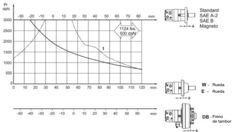
Diagrama de funciones MLHSBD
