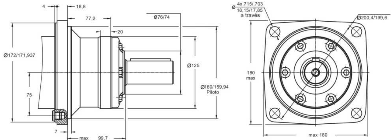
Versiónes 2, 3, 4, 5 Ejes laterales
