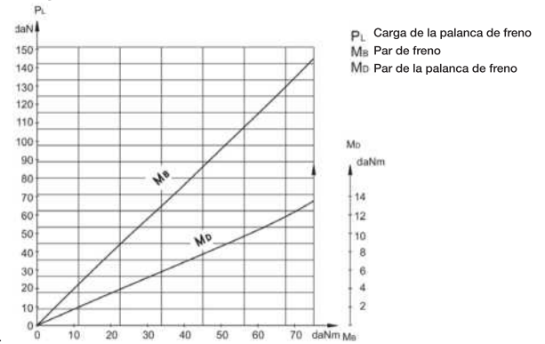
Diagrama de funciones MLHSBD
