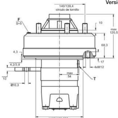
BD Brida Versiones 2, 3, 4, 5
