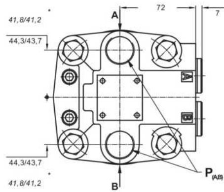
Versiónes 6, 7, 8, 9 Ejes traseros
