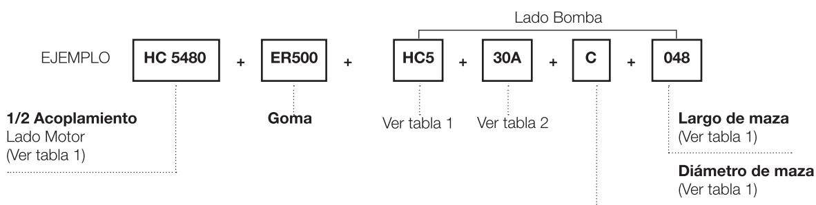
Código de maquinado lado bomba
